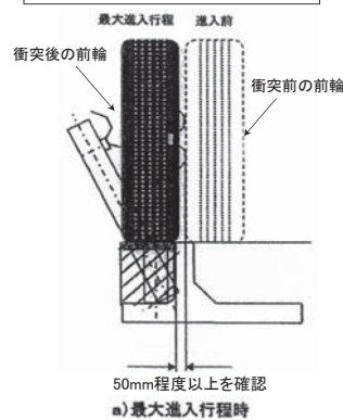
図 前輪が路面に残る幅の説明図
