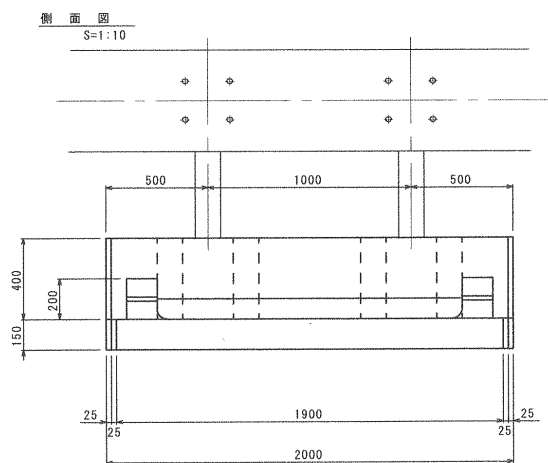
高速道路用プレガード (SB種用)
