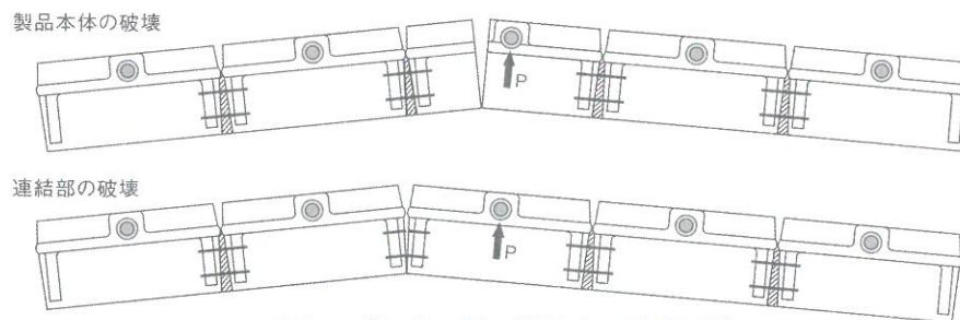
図-2 プレガードの縦方向の破壊形態
