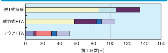
直工費と施工日数の比較(当社調べによる)
